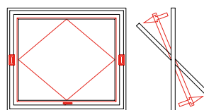
Ventana pivotante
