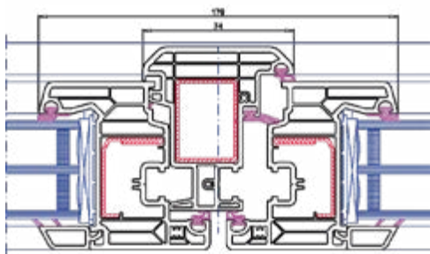
Sección central
